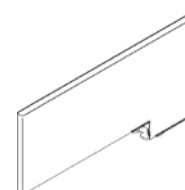
Écran latéral magnétique recouvert de tissu L 750 mm x H 305 mm
